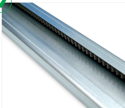
stabile Zahnriemen-Laufschiene für einen geräuscharmen und wartungsfreien Lauf
